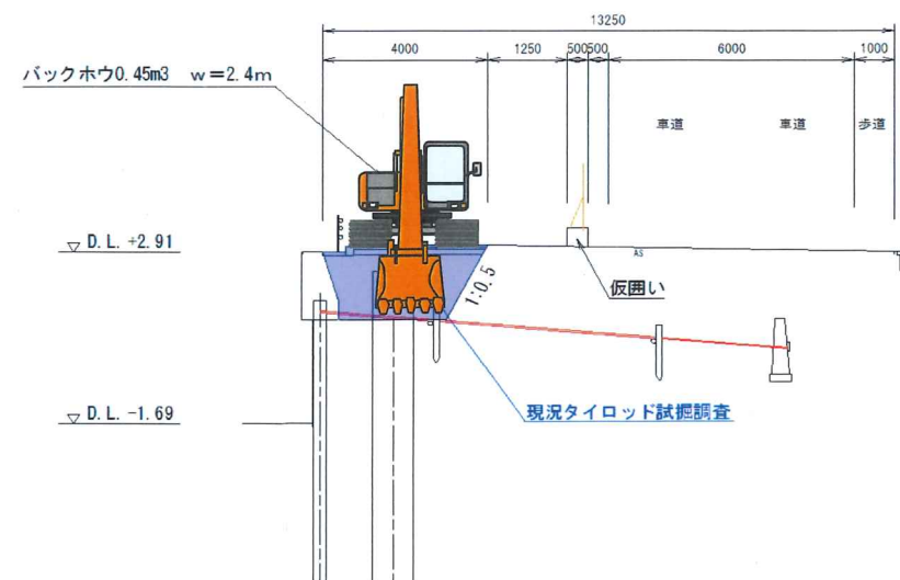
標準断面図
